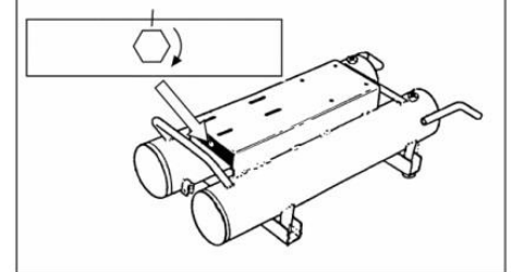
Figura 4 Girar el perno 1/2 pulgada en el sentido de las manecillas del reloj aumentará la tensión de la correa
