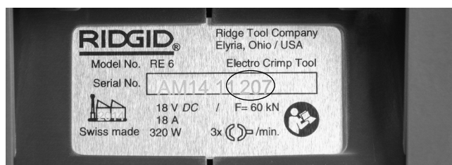
Figure 3 – Numéro de série de l'appareil – Les 4 premiers chiffres (encadrés) indiquent l'année et le mois de fabrication. (12 = année, 06 = mois).
