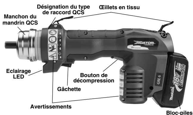
Figure 1 – Pinces électriques types RE 6 et RE 60 avec raccords rapides QCS pour le montage des têtes
