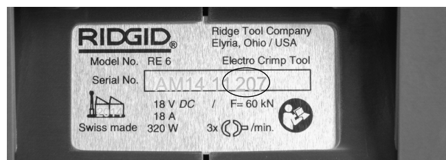
Figura 3 – Número de serie de la máquina. Los 4 dígitos iniciales (marcados con un círculo) indican el año y el mes de fabricación (12 = año, 06 = mes).
